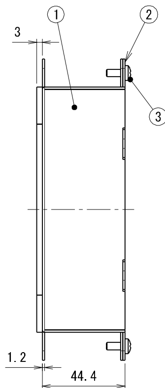
断面 A-A
