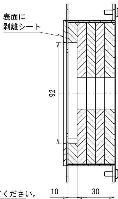
断面 A-A
