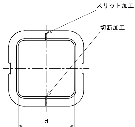
スリット加工図
