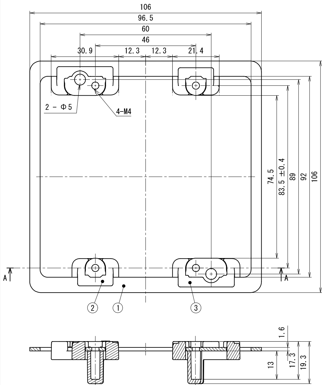
断面 A-A
