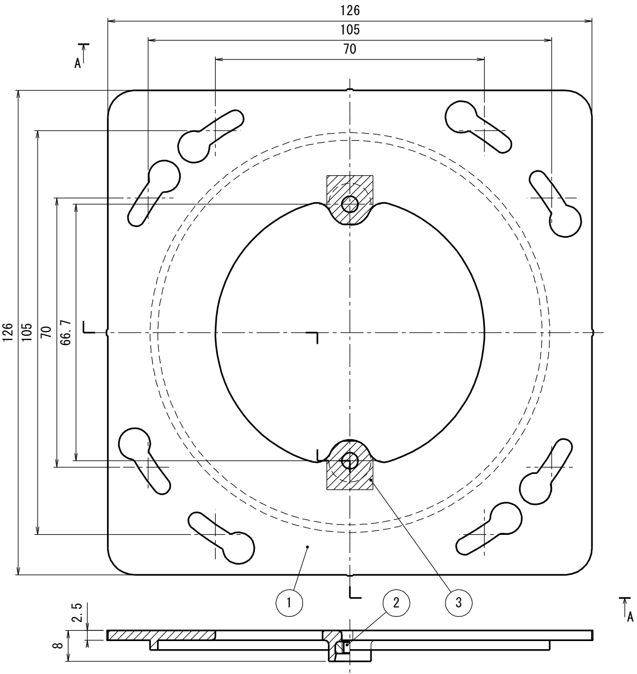
A-A断面図
