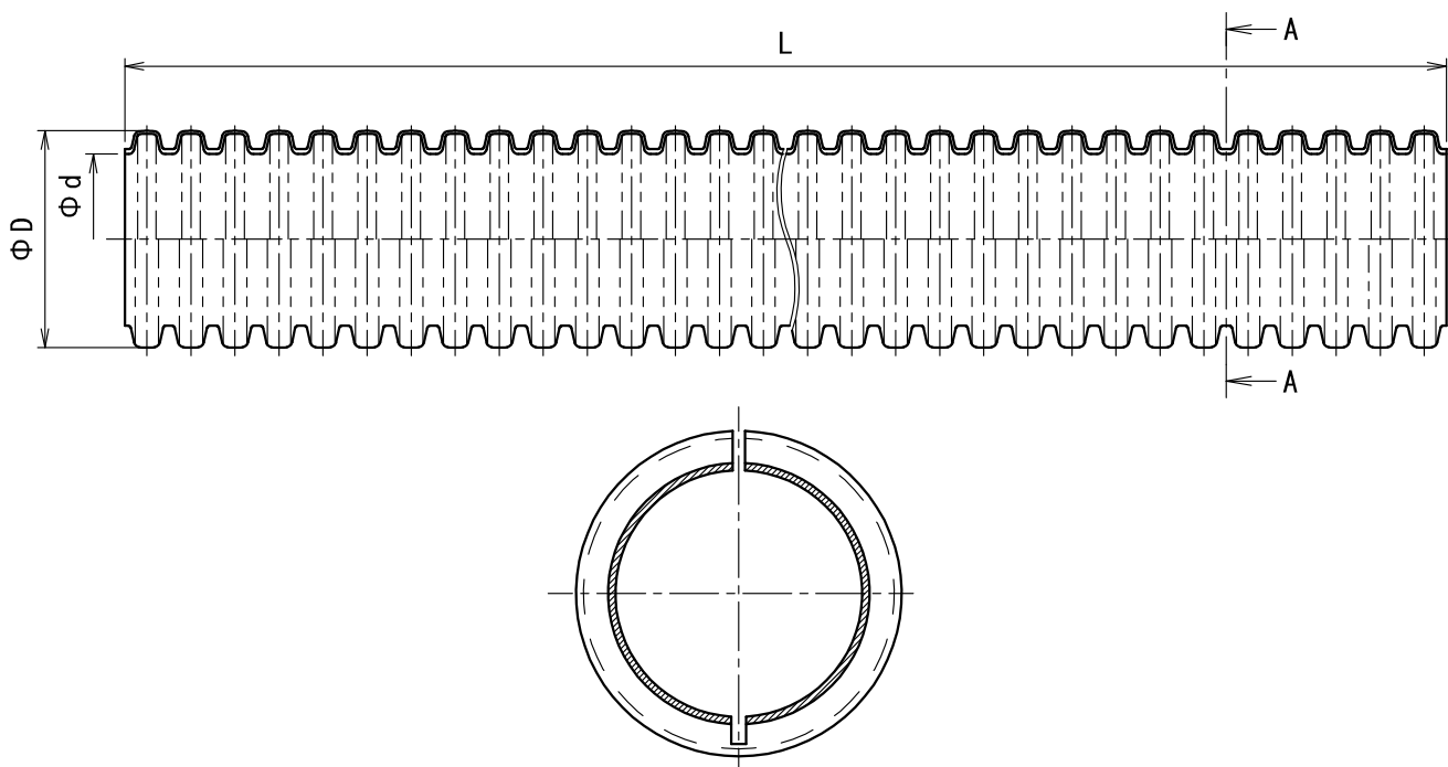
A-A断面図 (半割れタイプ)
