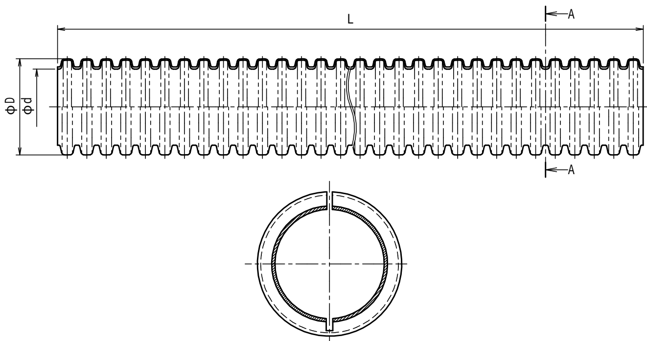
A-A断面図
