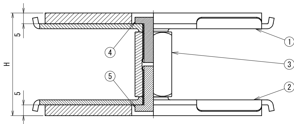
断面 A-A
