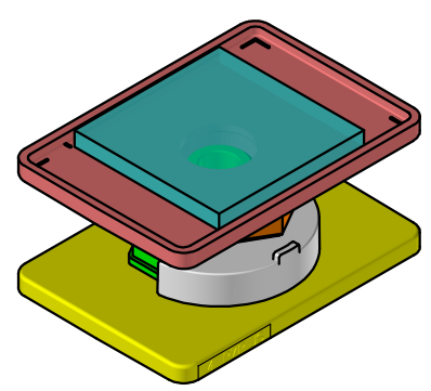
斜視図(組付状態)
