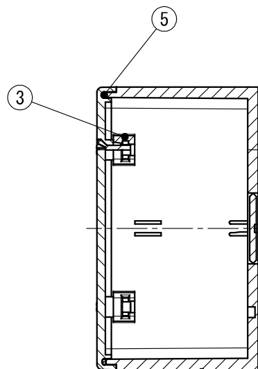
断面 A-A
