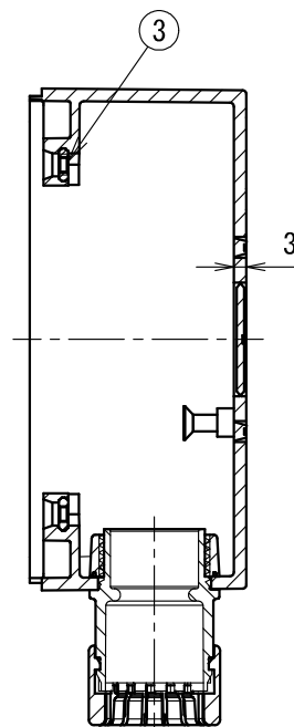
断面 A-A
