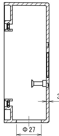
断面 A-A
