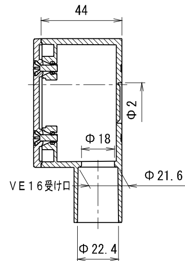
断面 A-A
