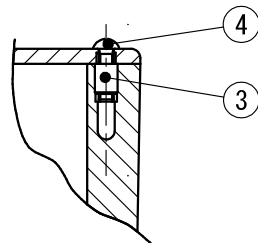
ねじ部詳細図 (1/2)
