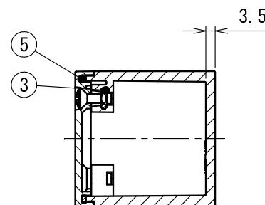
断面 A-A
