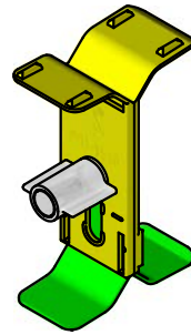
参考斜視図（1/3）
