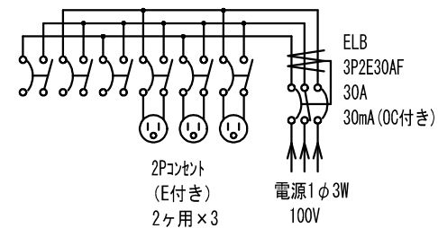
結線図
