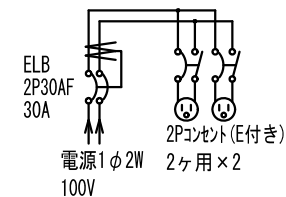
結線図
