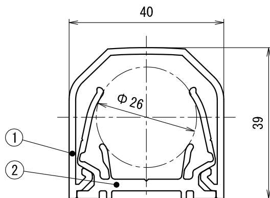
RMN-20_ (断熱材無し)
