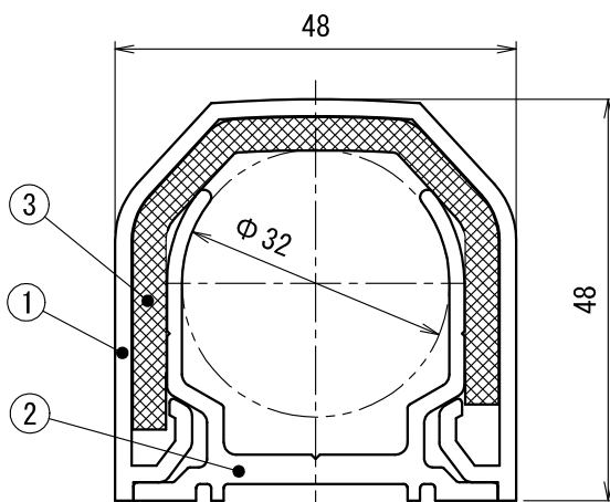
RM-25_ RMN-25_ (断熱材無し)
