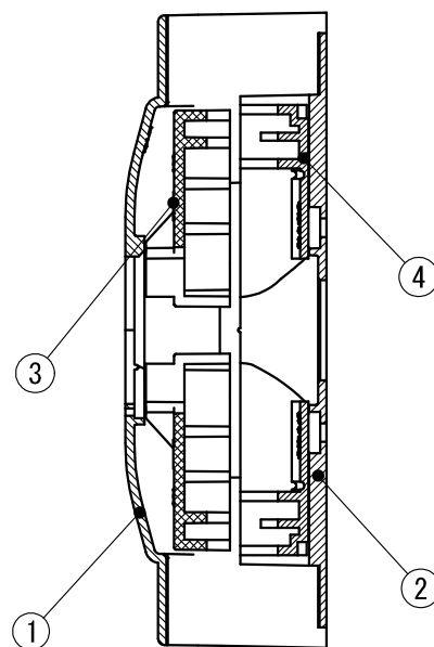
断面 A-A
