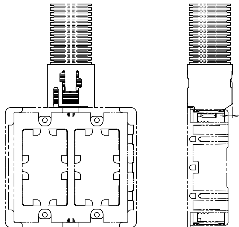
■組付け状態 (1:2)
