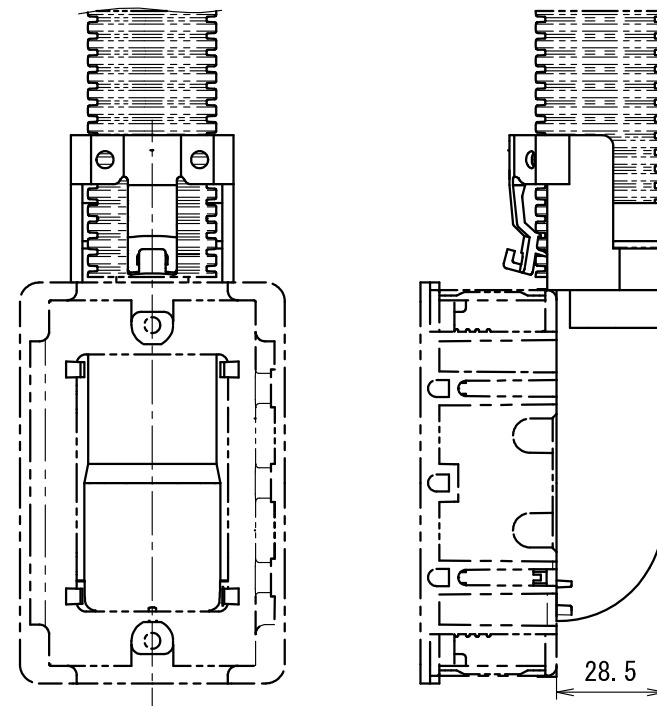
■組付け状態 (1/2)
