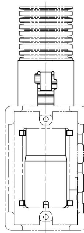
■組付け状態 (1:2)
