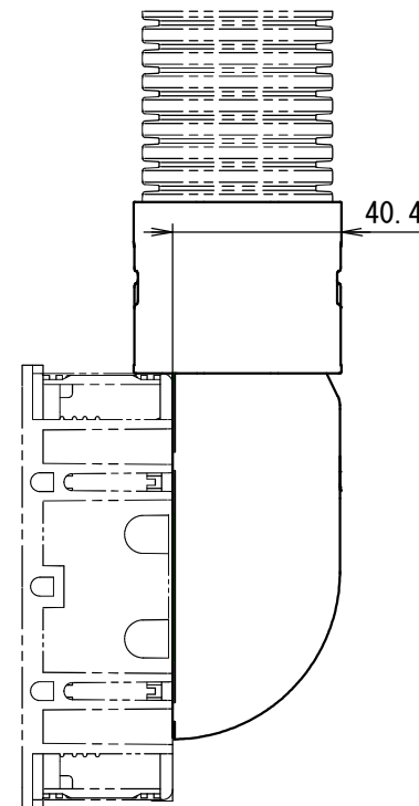
■組付け状態 (1:2)
