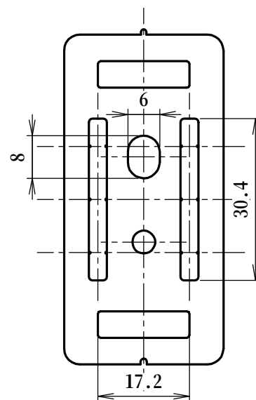
背面図
