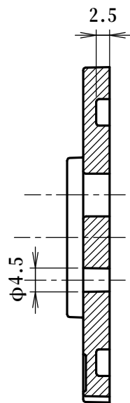
A-A断面図
