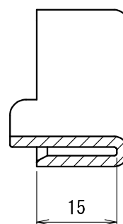
A-A断面図
