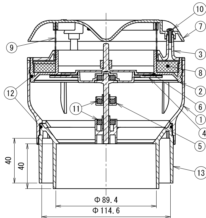
A-A断面図
