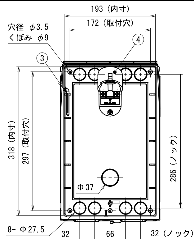
蓋無し参考図
