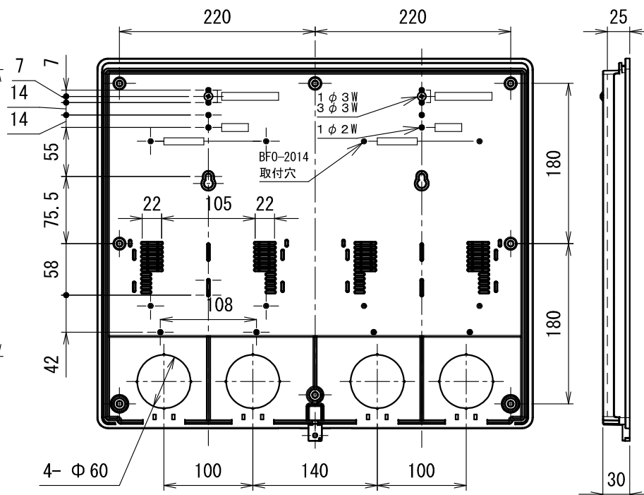
基台（取付板）
