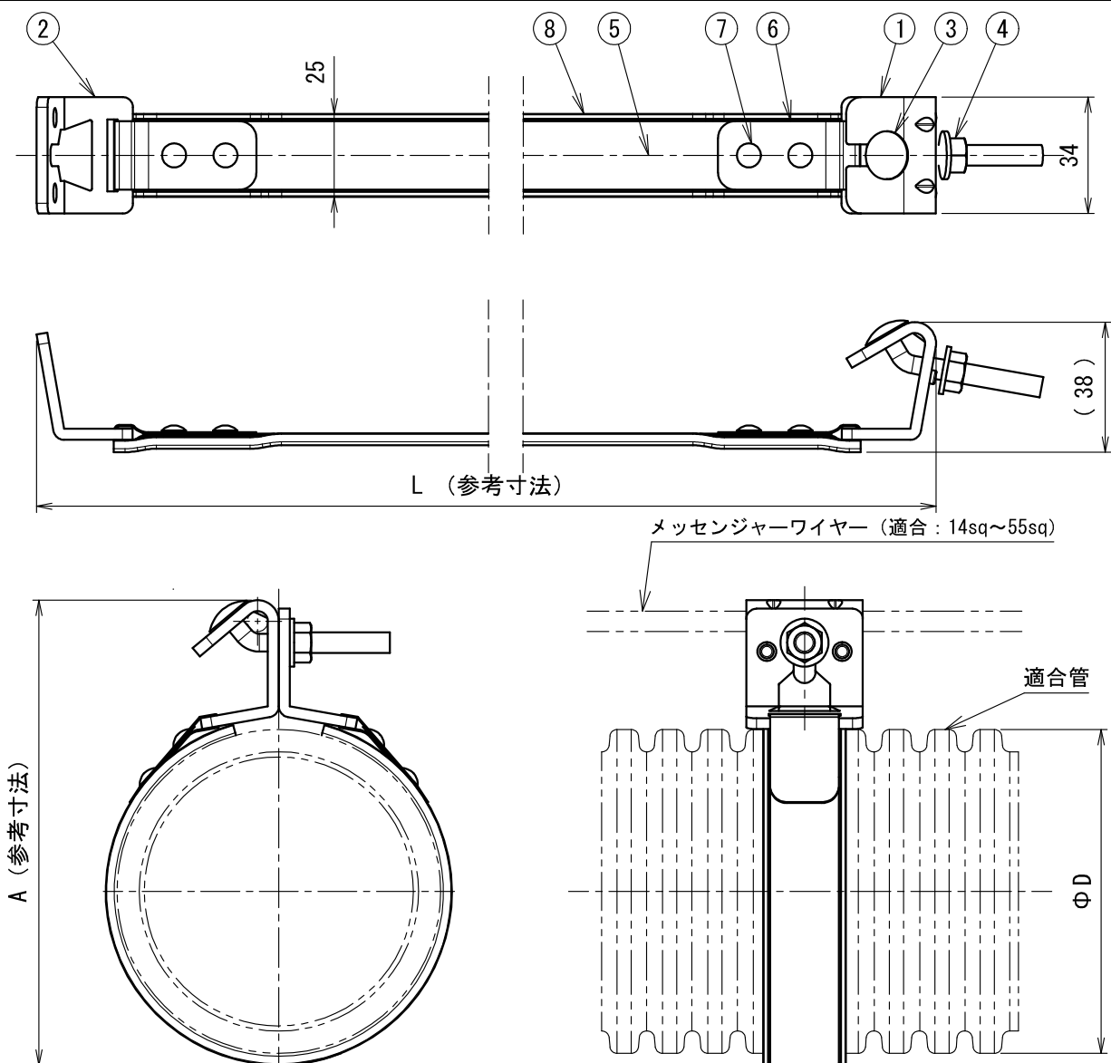
施工図
